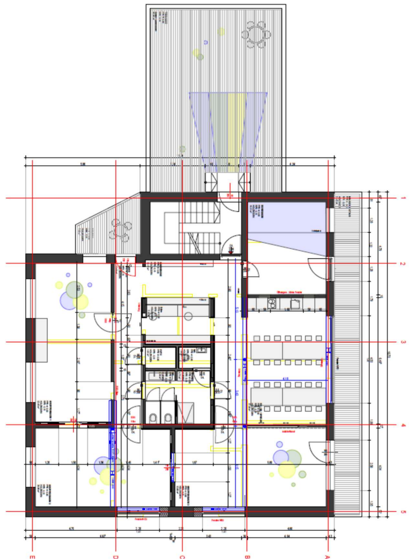
Raumplan
